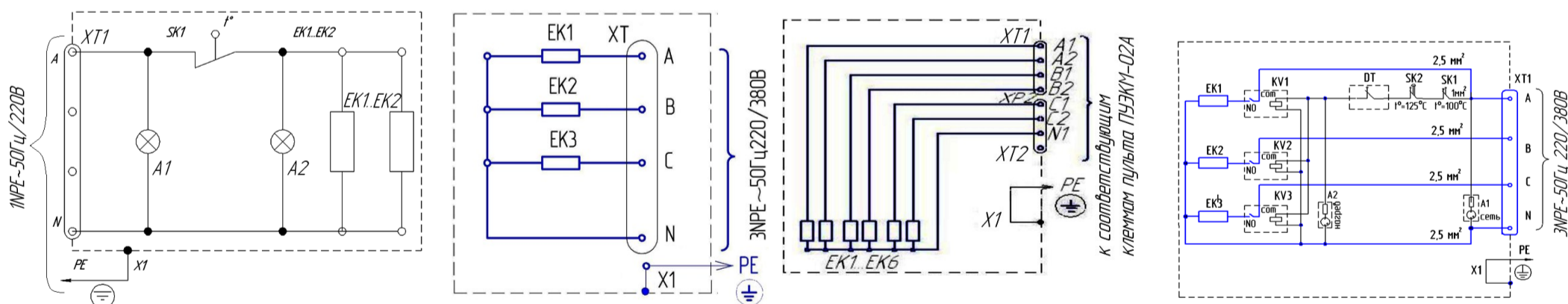
Рисунок 1 – Общие виды и устройство электрокаменок
